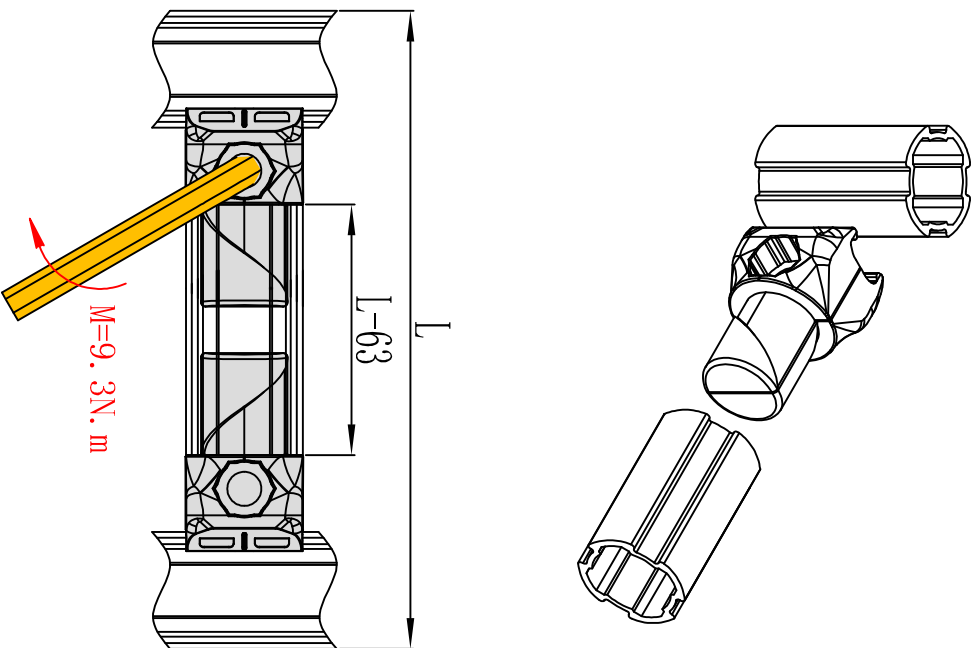
安装示意图
